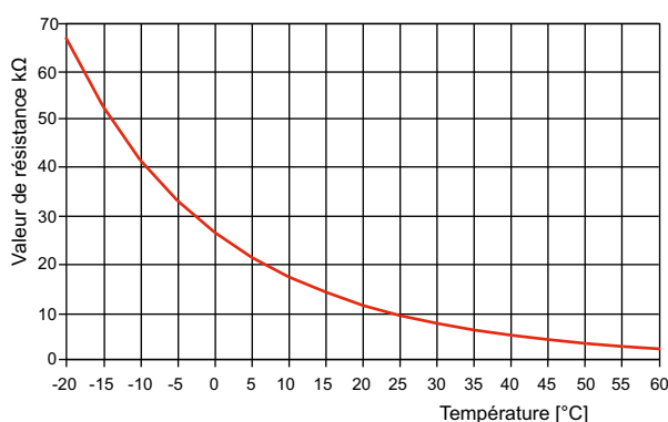
Fig. 7.1: Courbe caractéristique de la sonde NTC-10
